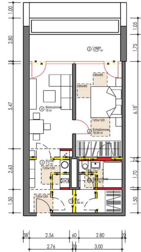
Konzept 1 Barrierefreie Wohnung
